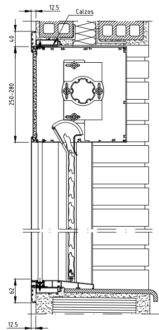
SECCIÓN VERTICAL (enrollamiento exterior)
