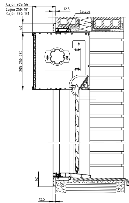
SECCIÓN VERTICAL (enrollamiento interior)
