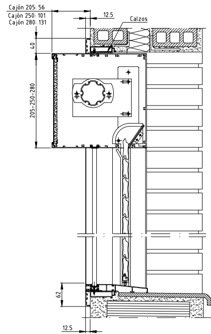
SECCIÓN VERTICAL (enrollamiento interior)
