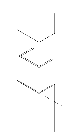
Detalle empalme. Marcos fachada vertical.
