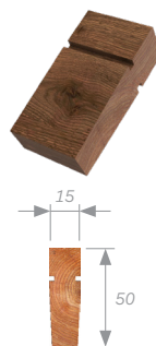
Thermopine Sección lamas (cotas en mm)
