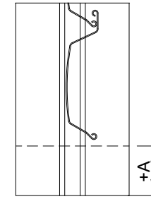
Solución guía prolongada para ajuste en obra
