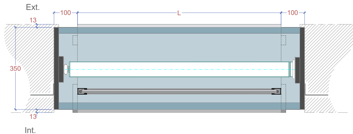
Enrollamiento Exterior
