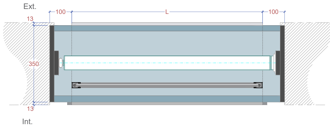
Enrollamiento Exterior
