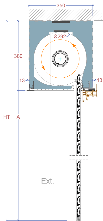
Enrollamiento Exterior
