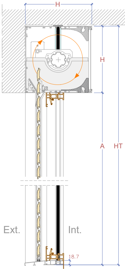
SECCIÓN VERTICAL Enrollamiento Interior
