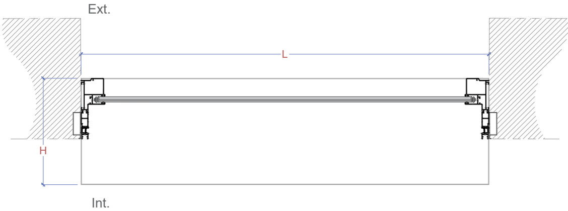
ENROLLAMIENTO INTERIOR Secc. planta Alucomplet Guías estándar 160
