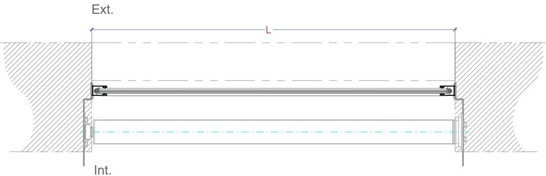
ENROLLAMIENTO INTERIOR Secc. planta con soporte incorporado en guías.
