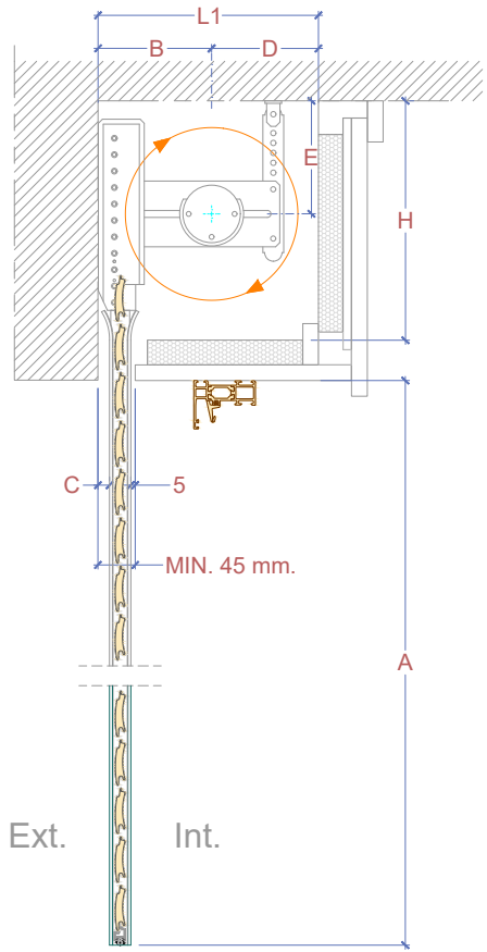
SECCIÓN VERTICAL Enrollamiento Interior Soporte incorporado en guías
